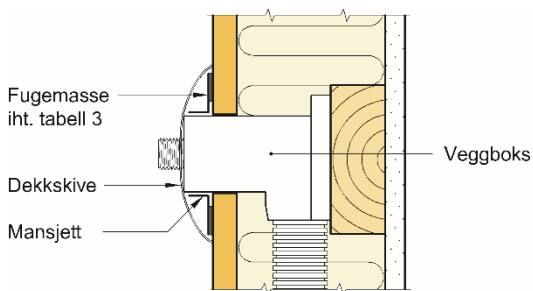
Figur 2 Rørgjennomføring hvor mansjett limes fast til Veggpanelet
