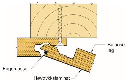
Figur 1 Fibo Veggpanel med Aqualock låsesystem
