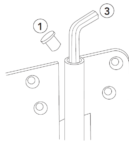
Fig 38. Høydejustering av hengsler gjøres med 5mm umbrakonøkkel.
