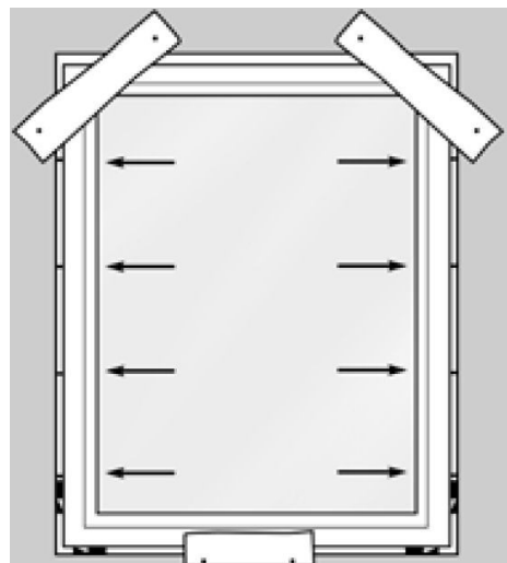
Fig 18. Samtlige hylser skal være løsnet ved montering
