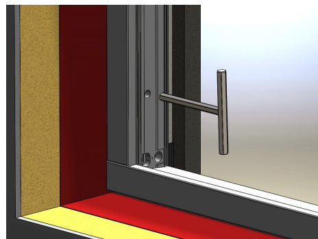
Fig 17. Slik skruer du ut karmhylsen
