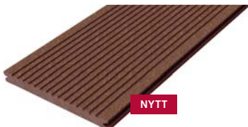
Barbentgulvet CLASSIC PLUS 21 × 242 mm (Jumbo) L: 300 / 360 / 420 / 480 / 540 / 600 cm
