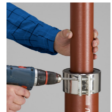
Elektrisk eller trykkluftskrutrekker kan benyttes.
