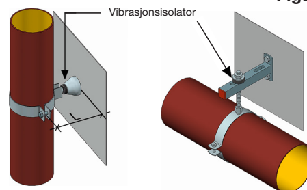
Figur 4.2. Opphengsløsninger for vibrasjonsisolerende rørfeste. Vertikalstamme, minimum 1 akustikkdemper pr 3 meter. Horisontalstamme, minimum 2 akustikkdemper pr 3 meter.
