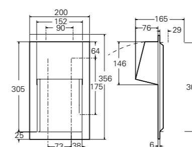
Easy ASI0031 Innfelt dobbel toalettullholder GTIN 4005683042855
