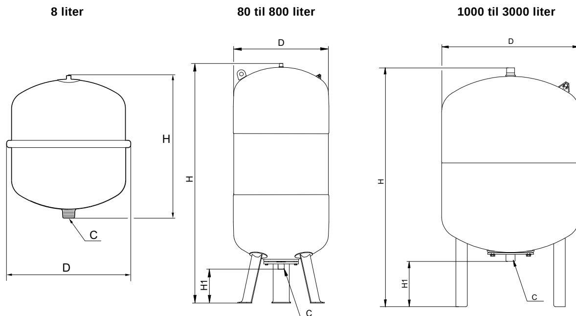
Fig. 8 Målkitser
