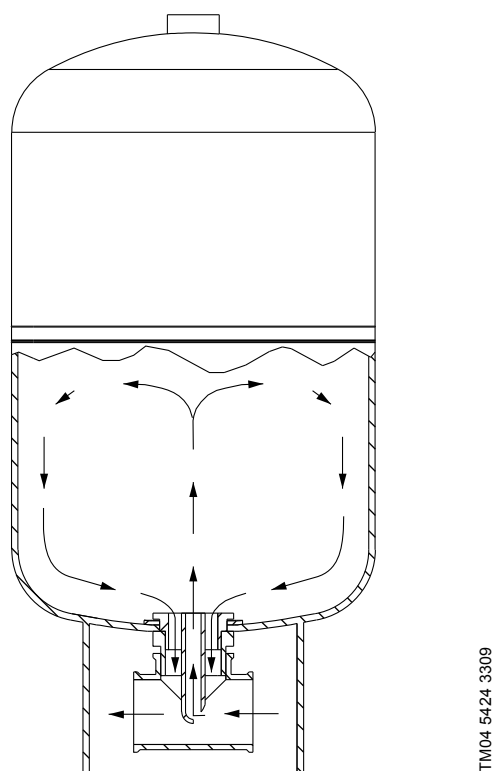
Fig. 3 Illustration af FlowThru-princippet
