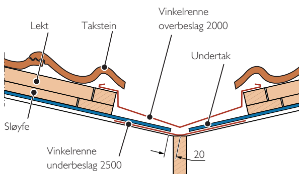
Detalj ved vinkelrenne.
