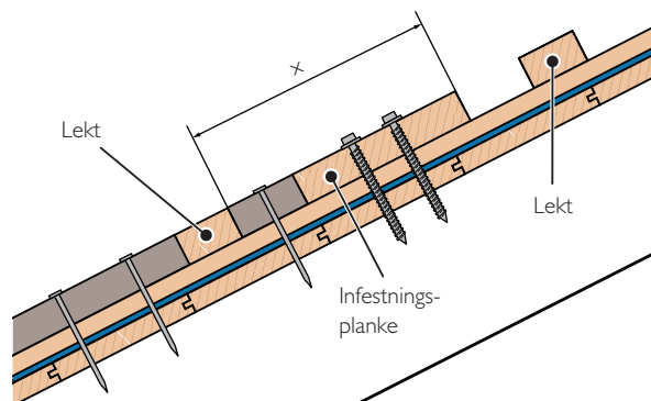
Innfestingsplanke.
