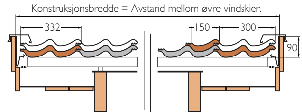
Konstruksjonsbredde uten bruk av gavlstein for Zanda betongtakstein..
