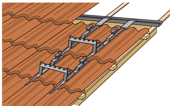
Feste taktrinn..
