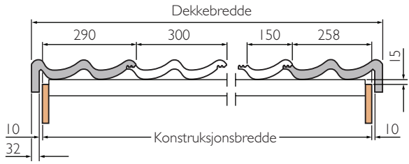
Bruk av gavlstener for Zanda betongtakstein.
