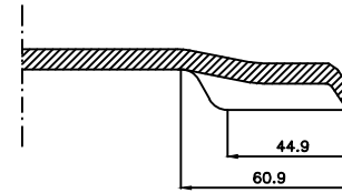
Snitt D-D
