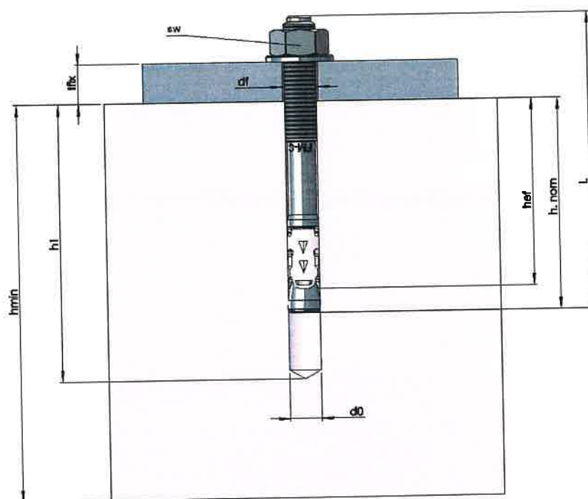
Figure A2: Installed MFT EKSPANSJONBOLT SYREFAST A4 OP.1 anchor
