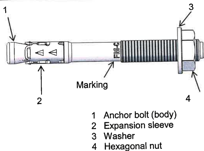
Figure A1: MFT EKSPANSJONBOLT SYREFAST A4 OP.1 anchor
