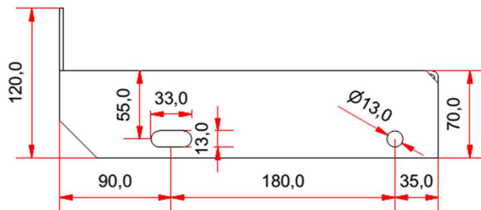
Tegning av endestykke for innskruing
