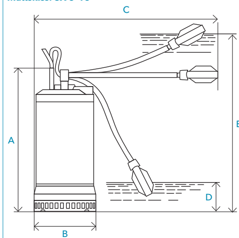
Måttkiss: SX 5-15
