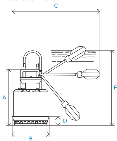
Måttkiss: SX 2-3
