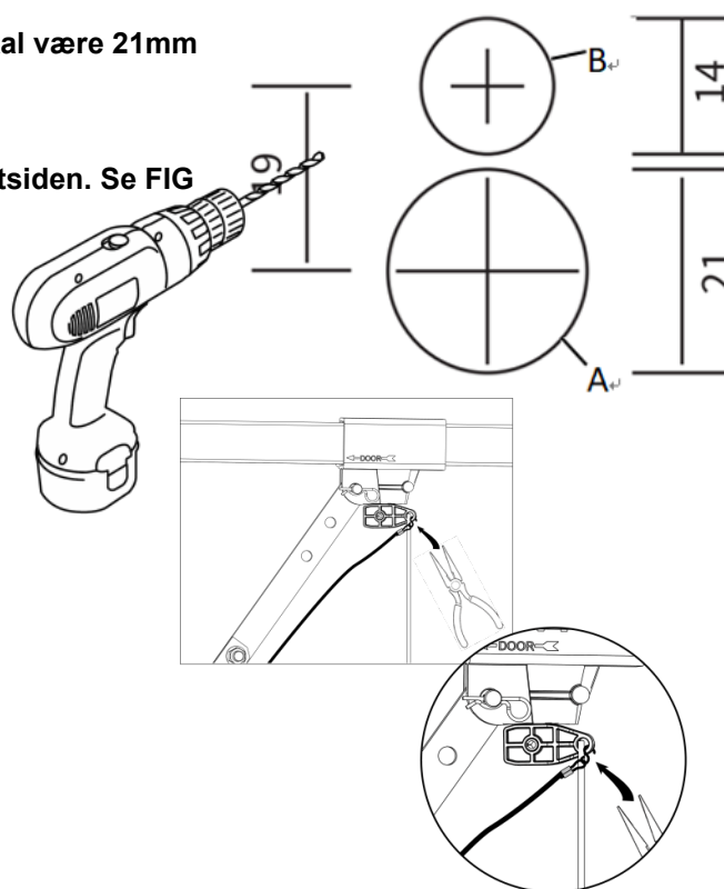
(Fig. 1 - Tegning for boring av hull)
