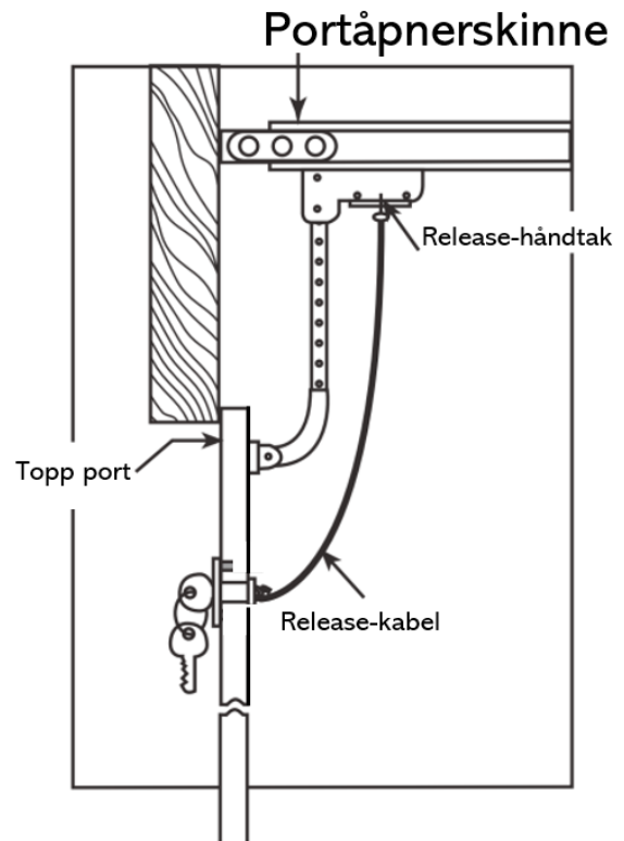
(Fig. 2 - Tegning for boring av hull og bruk)
