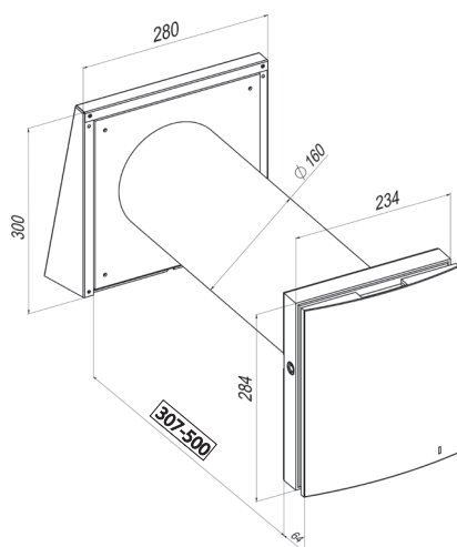
Byggemål innendørsenhet [mm]
