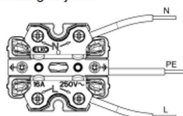
Koblingskjema
