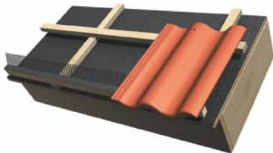
Bilde 9. Fuglebåndet monteres på takfotslekten. (Takfotslekten skal være 10 mm høyere enn bærelekten.) Se bilde 2 og avsnitt "Lekting". Ved bruk av ventilert fuglebånd har dette en byggehøyde på 25 mm.
