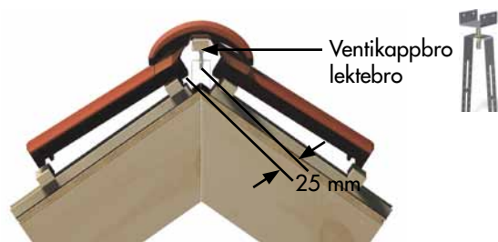
Bilde 3. Som mønekam kan du med fordel bruke ventikapp lektribro. Den er justerbar og kan bygges opp til riktig høyde med en lekt. Bredden får ikke overstige 36 mm.
