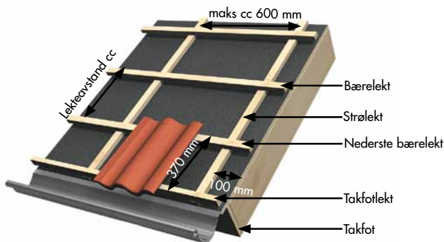
Bilde 2. Lekteavstand måles fra overkant til overkant. Merk at målet på første bærelekt er fra nedkant takfot til overkant første bærelekt. Dette målet er 370 mm. Takfotslekten må også være ca 10 mm høyere enn de andre lektene fordi nederste takstein ikke hviler på noen taksteinsrad. (gjelder ikke ved bruk av ventilert fuglebånd.)
