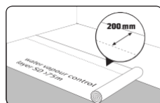
Underlag legges med 200 mm overlapp
