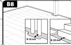
Avstand til rør og faste installasjoner som f.eks trapp
