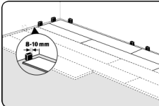
Avstand til vegg (8-10 mm)
