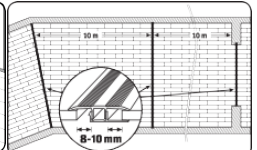
Maks lengde / bredde: 10 m samt bruk av overgangslist
