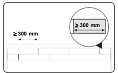
Endeforskyvning og siste bord pr rad (Woodstock XL min 500 mm forskyvning)
