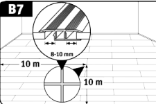
Maks areal / lengde og bredde og bruk av overgangslist
