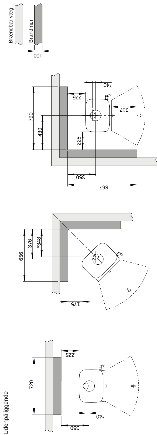
Jøtul F 105 R Min. afstand til brænbar væg beskyttet af godkend brandmur
