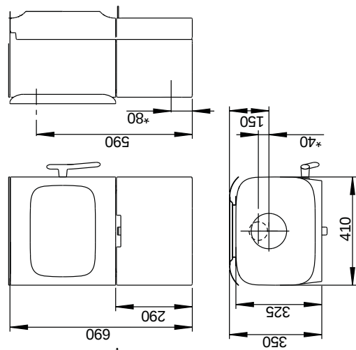
Jøtul F 105 med sokkel
