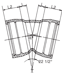
S-9175 Tyton bend 22 1/2° Med to muffer
