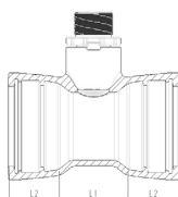
S-9121 Dobbeltmuffe m/Esco Lock* Bajonettkobling i avsinkningsfri messing Med 2 " utv og 1 1/2 innvendige rørgjenger
