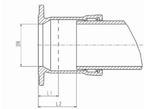
S-9170-4 Flensemuffe
