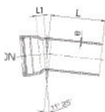
S-9674 Muffespiss bend 11 1/4°
