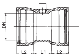
S-9171-4 Dobbeltmuffe
