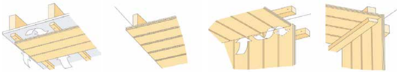
Spikerslag som sikrer luftning.
