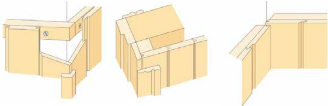
Stående panel skal først monteres på hjørner som vender utover, når slike finnes. Ellers begynner man i hjørner som vender innover. Begynn ved et hjørne og gå fra venstre mot høyre, snu notkanten mot høyre hvis du bruker spikerpistol. Husk å kontrollere med vater med jevne mellomrom.
