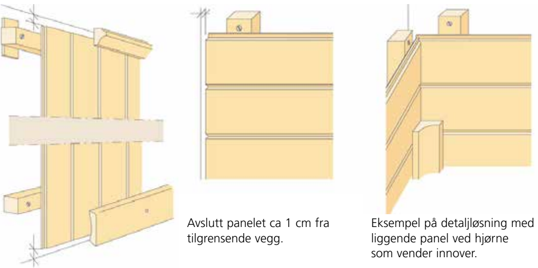
Avslutt panelet ca 1 cm fra taket og fra gulvet, og dekk dette med taklist/gulvlist.
