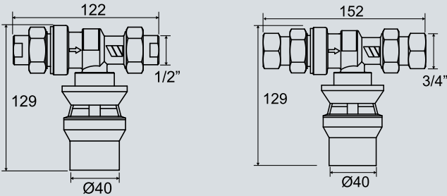
Tilbakeslagssikring 1/2"
