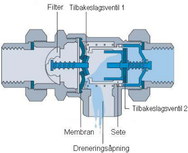
Ventilens innvendige komponenter
