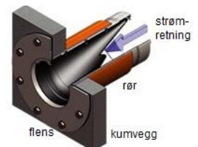
Montering på utløp vha flens
