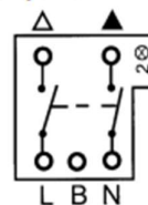
Koblingsskjema
