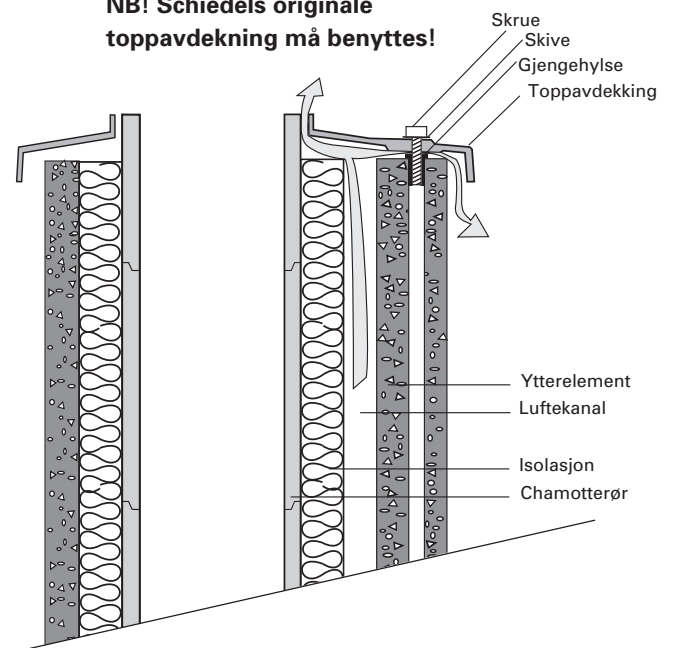
Pipetopp-utførelse Rondo
