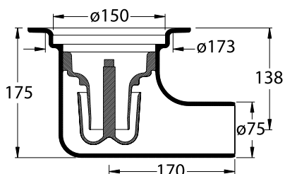
Tilfluktsromsluk
