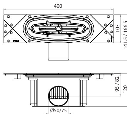
Sideutløp Ø50/75
