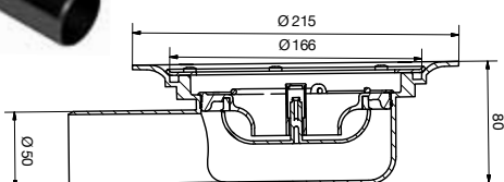
Lavbyggende sluk
