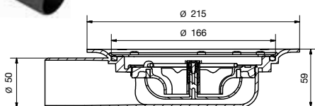
Lavbyggende sluk
