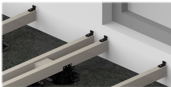
Figur 15: Monter brettet på underkonstruksjonen og trykk klipsene inn i holderne.
