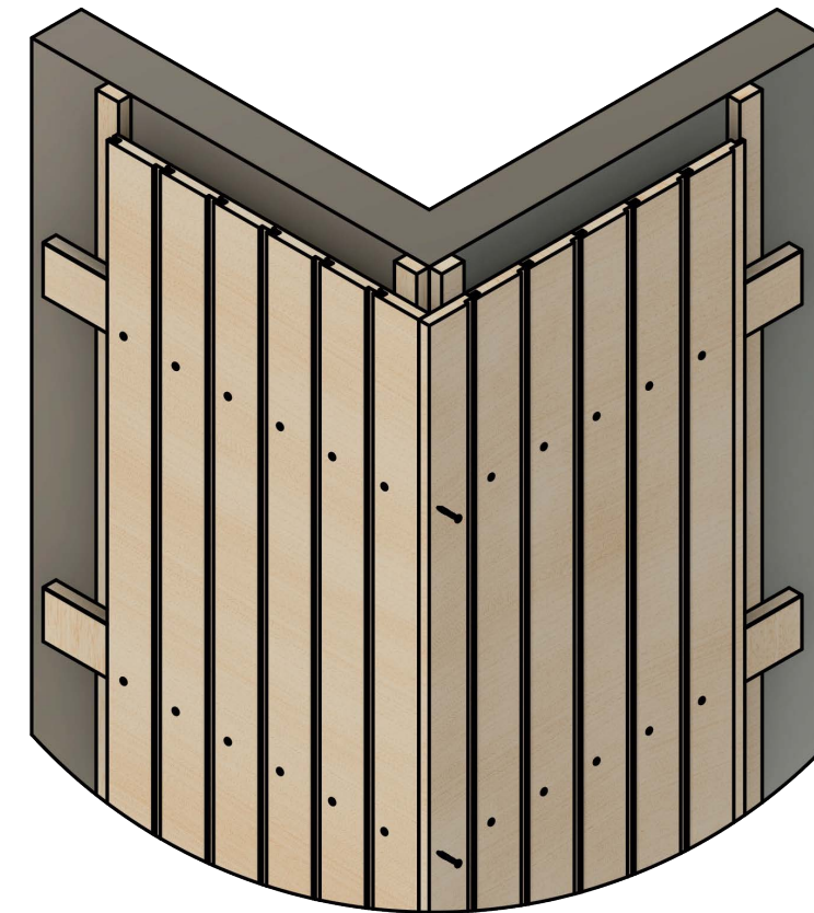
Figur 2: Hjørnedetalj
