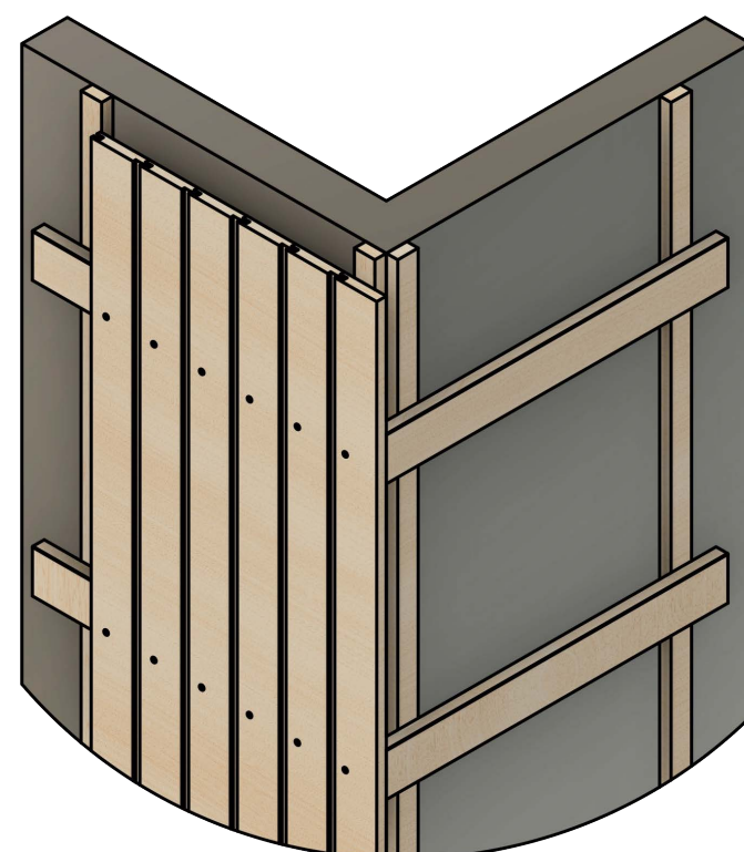
Figur 6: Hjørnedetalj
