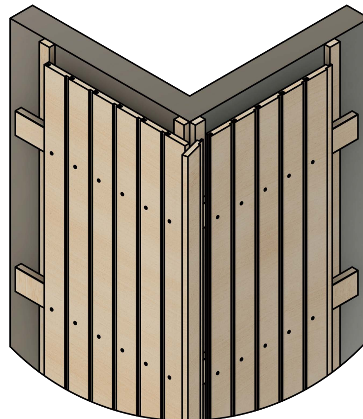
Figur 3: Hjørnedetalj
