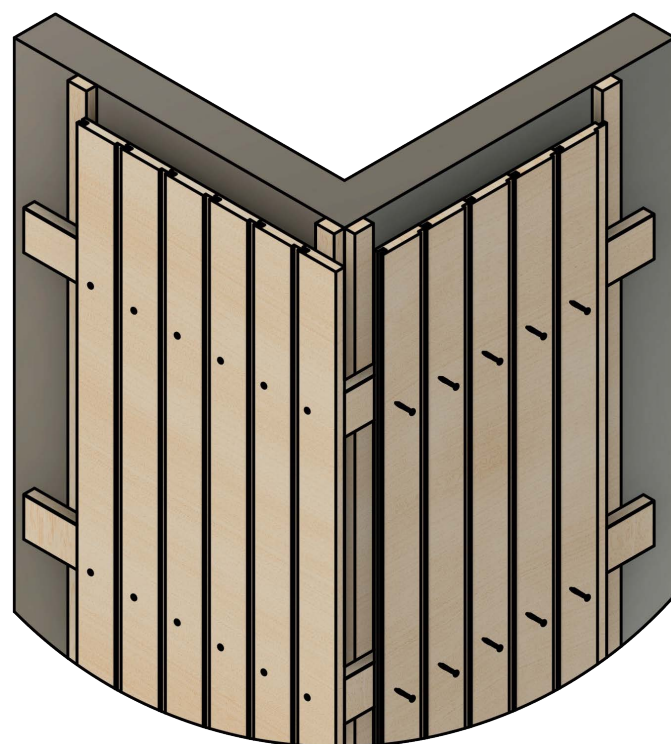
Figur 5: Hjørnedetalj
