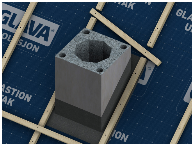
Fig. 20 Prinsipp for tetting rundt pipe, takhatt o.l. Unngå skjøter i duken ved gjennomføringen.
