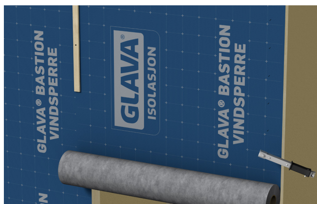
Fig. 35 Vertikal montering av vindsperre
