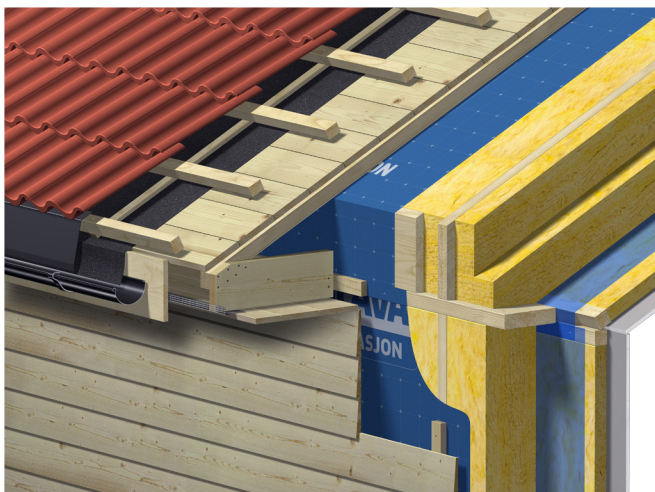
Fig. 33 Bastion vindsperre i takkonstruksjon med tradisjonelt lufteskikt
