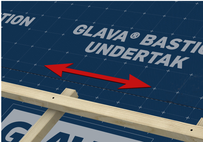
Fig. 9 Utstryking av omlegg
