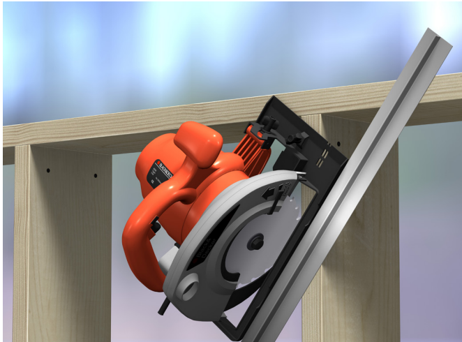
Fig. 30 Slissing i stenderverk for avstivningsstag
