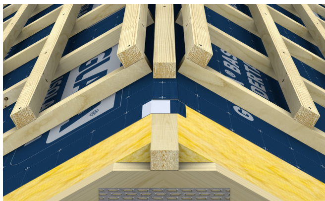
Fig. 17 Prinsipp for avslutning i mønet
