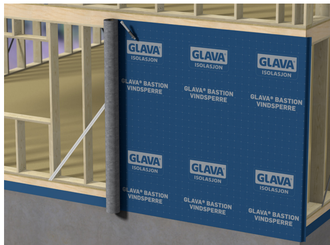
Fig. 34 Montering av etasjehøy vindsperre
