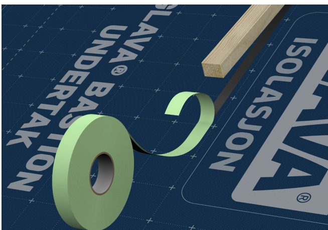
Fig. 6 Glava Dobbeltssidig butyltettebånd under sløyfer
