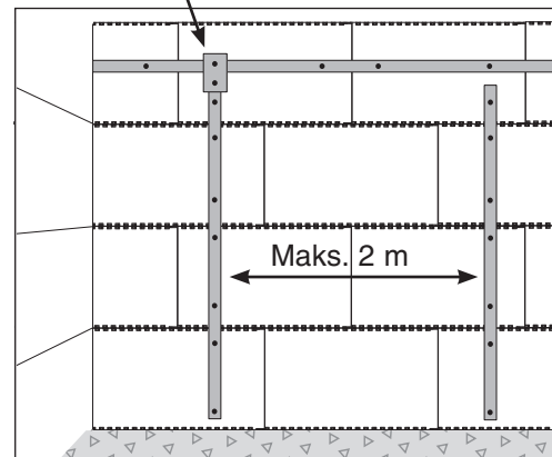
Sammenføyningsfeste
