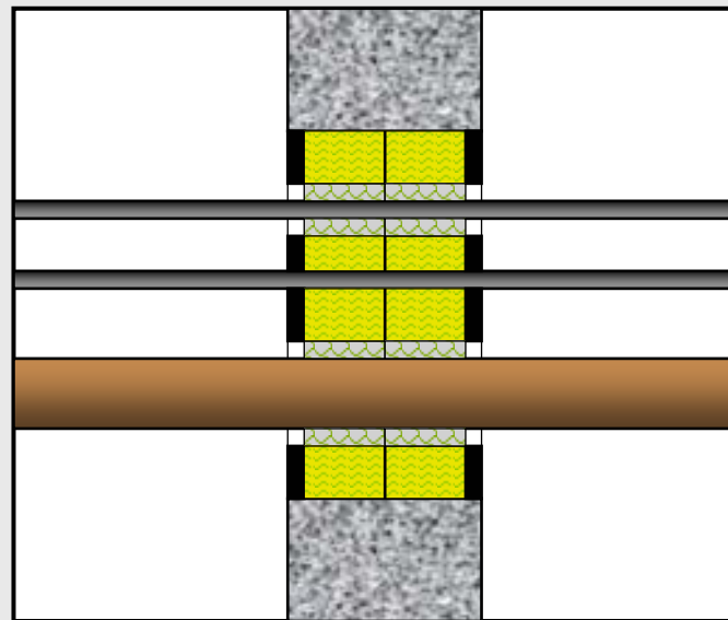
Betongvegg EI 60
