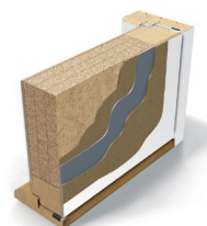
Innerdør EI30/35dB med klimastamme
