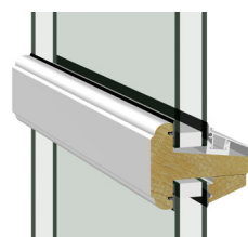
GJENNOMGÅENDE HORIZONTAL SPROSSE s/EE ↗
