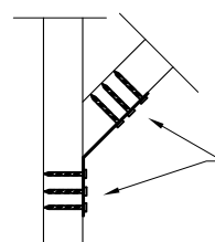
Snitt B-B
