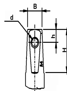
Dimensjoner spindeltopp:
