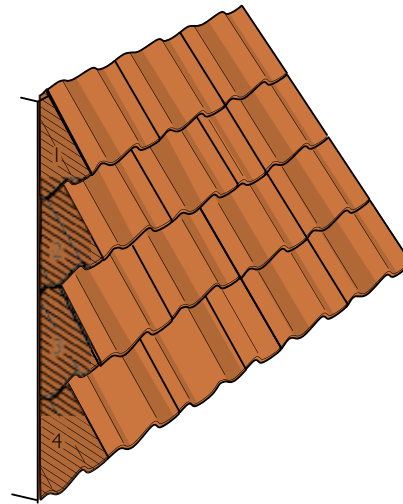
Figur 12: De kappede steinene forskyves til vinkelrennen når resten av steinene er lagt.
