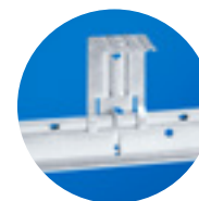
Justerbara pendlar och direktfästen (se nr 5, 7 på skiss nedan)
