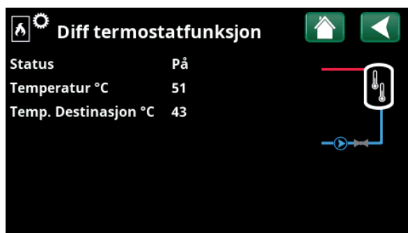
Meny «Driftsinfo/Difftermostatfunksjon».
