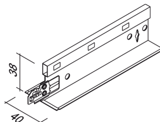
Tvärskena DXSF 120/90/60 med DONN DX Clip-Fix
