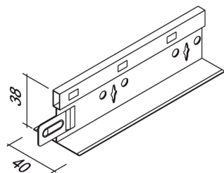
Bärskena DXSF 370 med änddetalj
