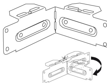
Modifierat beslag DCSC 180 för hörnlösning
