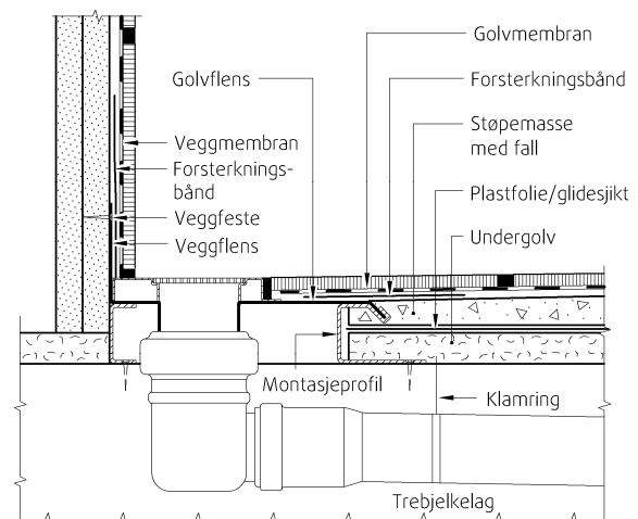
Fig 3 Unidrain gulvavløpsystem ved bruk av Unidrain montasjeprofil.
