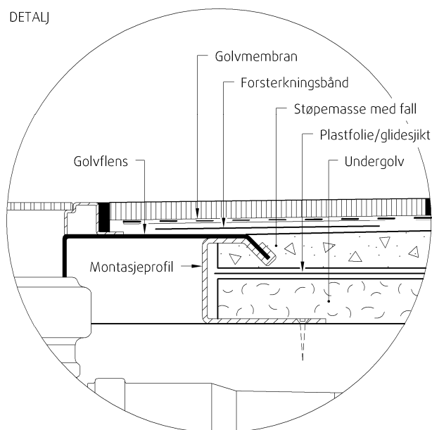
Fig 4 Detaljtegning. Overgang mellom sluk og golv.
