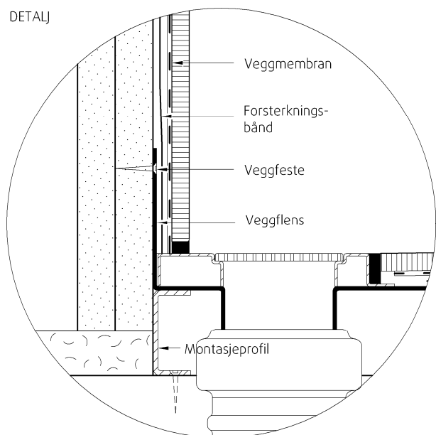
Fig 5 Detaljtegning. Overgang mellom sluk og vegg.
