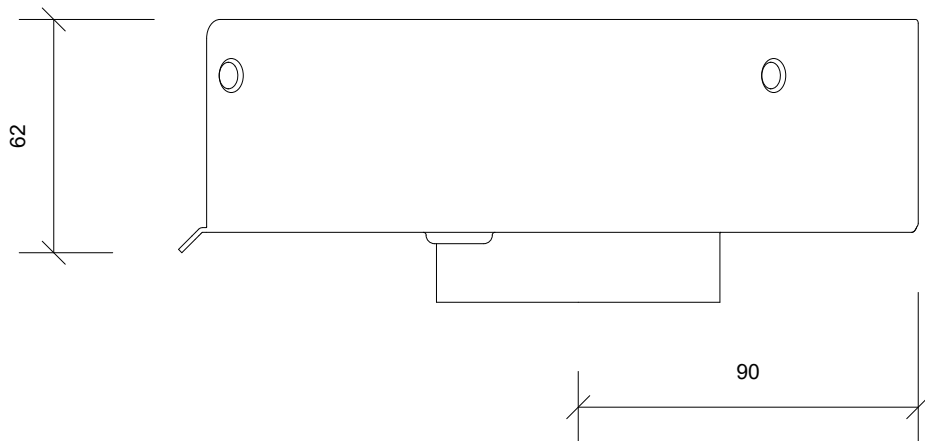
Side Opstalt/Side Elevation/Seitenansicht
