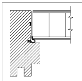
Profil av B30/25dB dør
