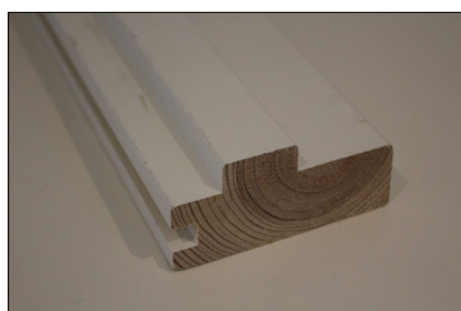
Snitt av standard 92 mm karm NB! Bildet viser ikke brannstrips. Denne er montert.
