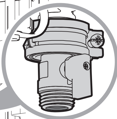
Tilkobling: kaldtvannstilførsel 3/4" utvendig gjenge
