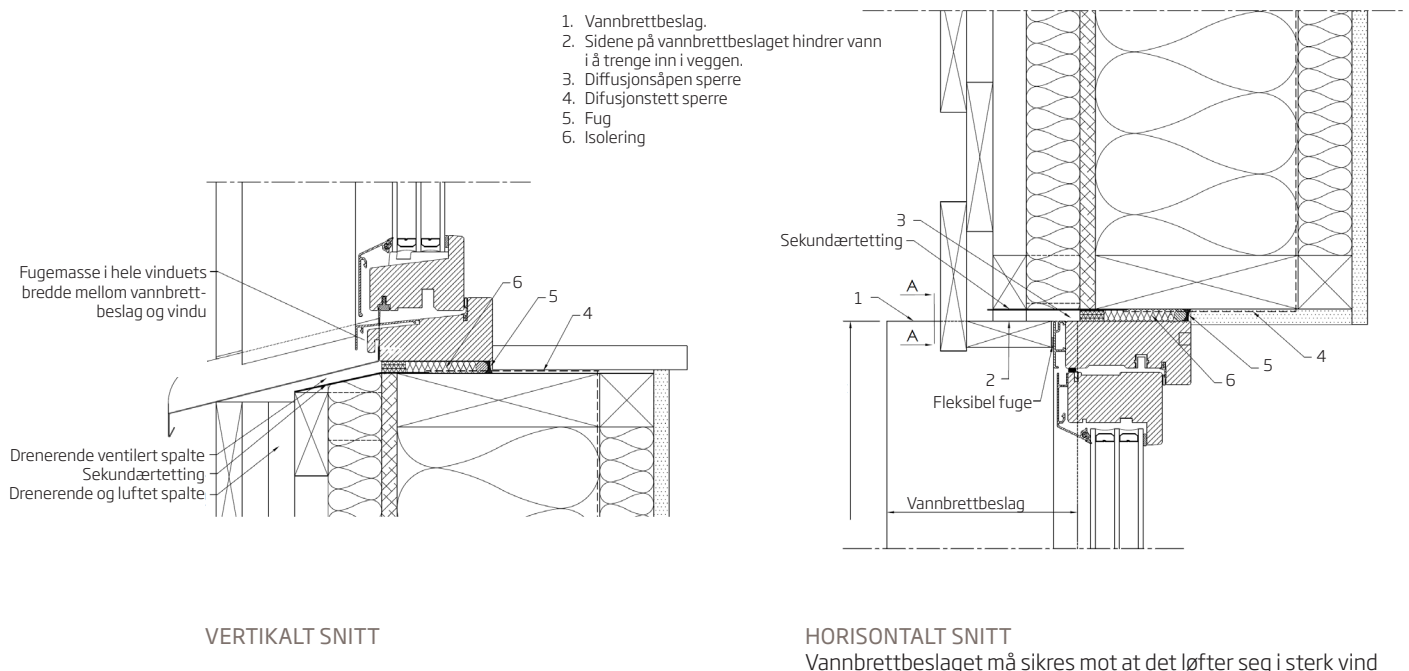
Fig 3. Snittet viser komponenter i vindusmonteringen. Det er viktig at den trykkutjevne spalten er ventilert og drenerende via sekundærtettingen for å unngå at fuktighet samler seg inne i vegg.
