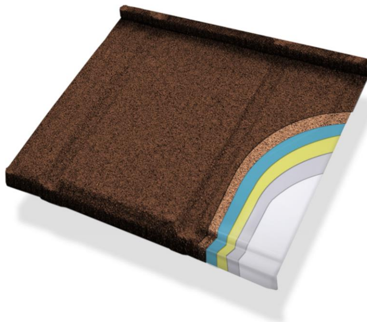
Figur 1, oppbygning av AeroDek Robust Plus
