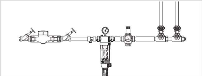
Monteringseksempel
