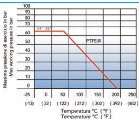
Trykk-/temperatur diagram for ikke-aggressive medier
