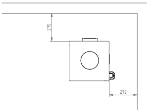
Afstand til brændbart med isoleret rørør
