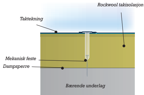
Prinsippskisse av kompakt, varmt tak
