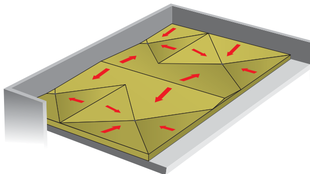
4-veisfall 1:40 og 1:60
