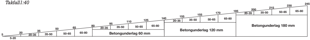
Takfall 1:40
