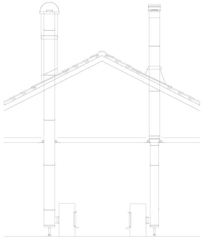
Baktilkoblet Helisolert
