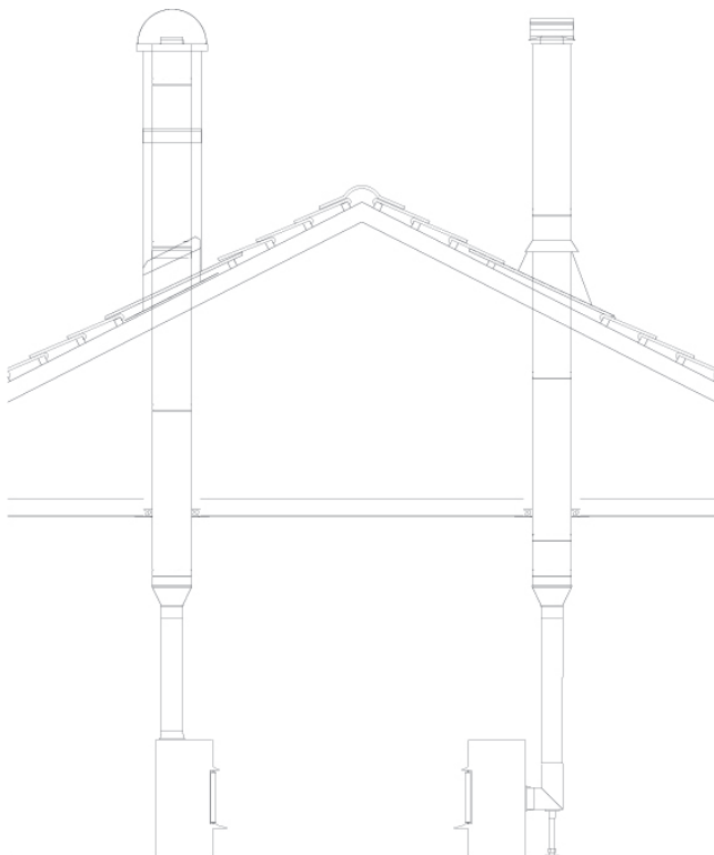
Topptilkoblet Uisolert
