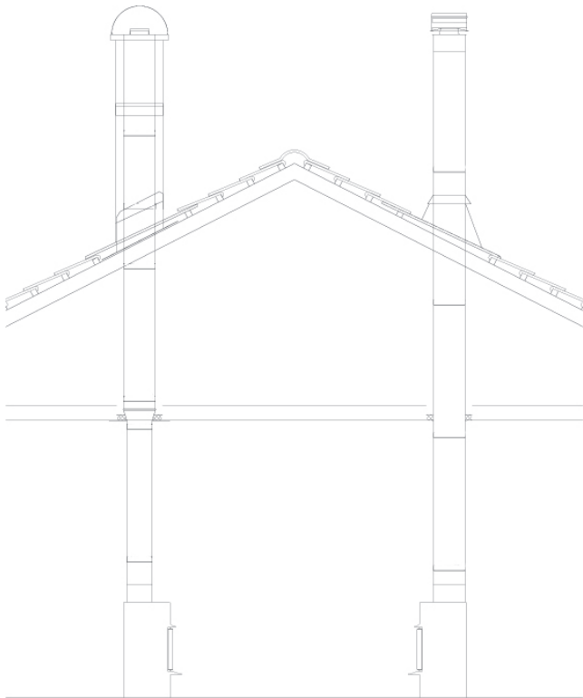
Topptilkoblet Halvisolert
