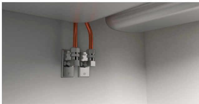
Når gjennomføring av LK PE-X og PAL Universalrør RiR uten veggboкс skal kobles til f.eks. kjøkken- eller vaskeromskraner, skal vinkelen på overgangen mellom LK PE-X - LK PAL-rør og blanderens rørforbindelse fikseres. Dette skjer forslagsvis med platealbu/ventilfeste.
