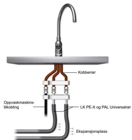
Åkseptabel løsning ved installasjon av kjøkkenarmatur med tilkoblingsrør av kobber med LK PE-X og PAL Universalrør RiR.
