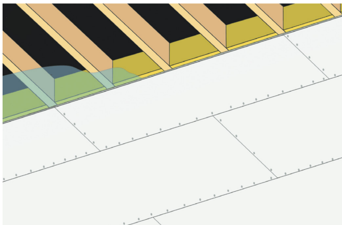
Illustrasjon for tak, se monteringsanvisning side 2
