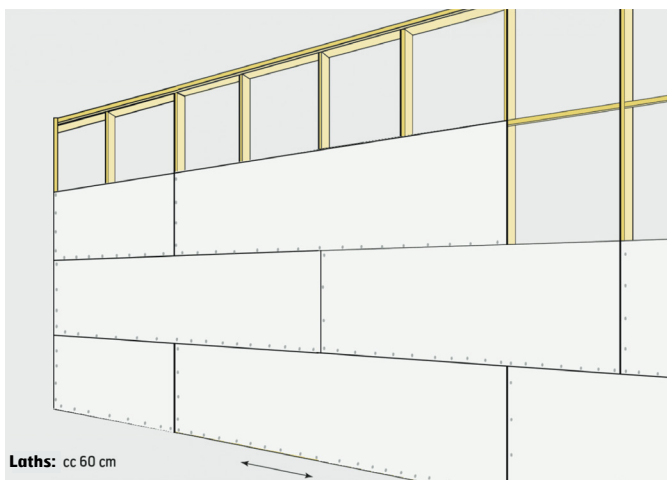
Illustrasjon for vegg, se monteringsanvisning side 3
